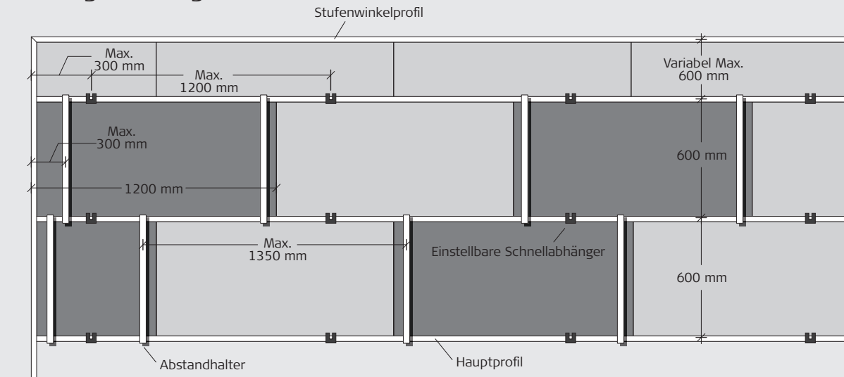
Abbildung – Montage
