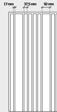
Troldekt® Line Design 11, 3/9 (ohne Nut 3 und 9)
