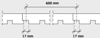
Modul, Breite
