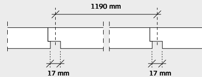
Modul, Länge
