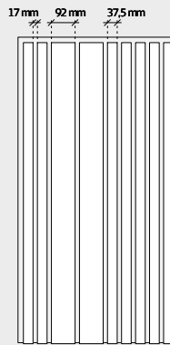
Troldekt® Line Design 11, 4/6 (ohne Nut 4 und 6)
