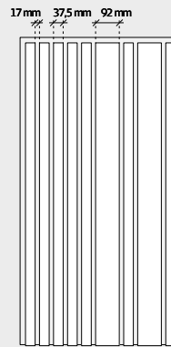
Troldekt® Line Design 11, 7/10 (ohne Nut 7 und 10)
