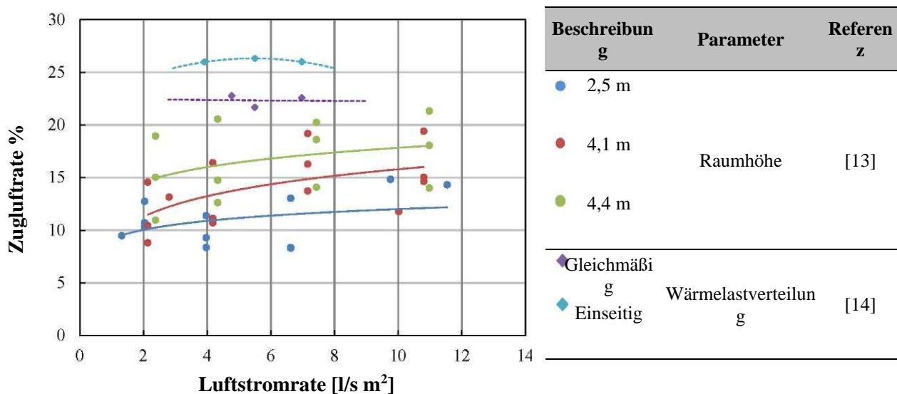
Abbildung 6: Zugluft im Verhältnis zur Luftstromrate bei verschiedenen Auslegungsparametern
