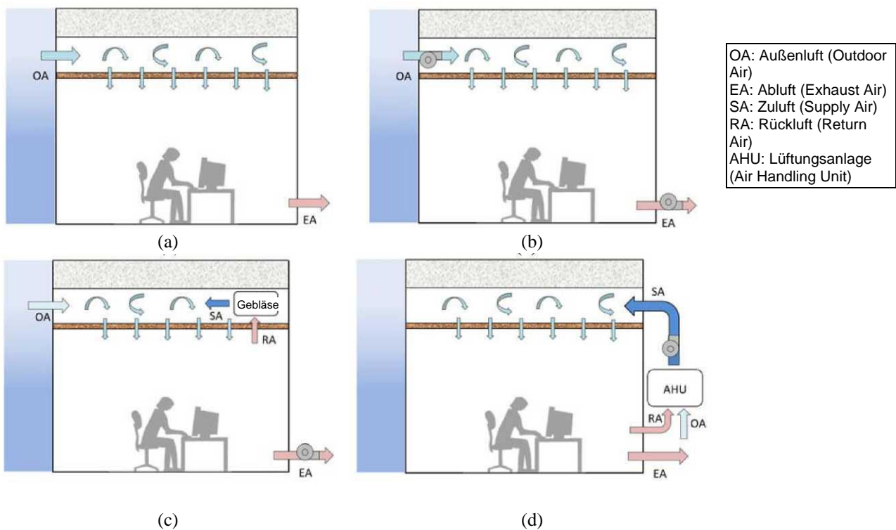
Abbildung 5: Schematische Darstellung verschiedener Lüftungsstrategien. (a) Natürliche Belüftung, (b) mechanische Lüftung, (c) hybride Lüftung mit Gebläsekonvektor, (d) Voll-kli-ma-ti-sie-rung
