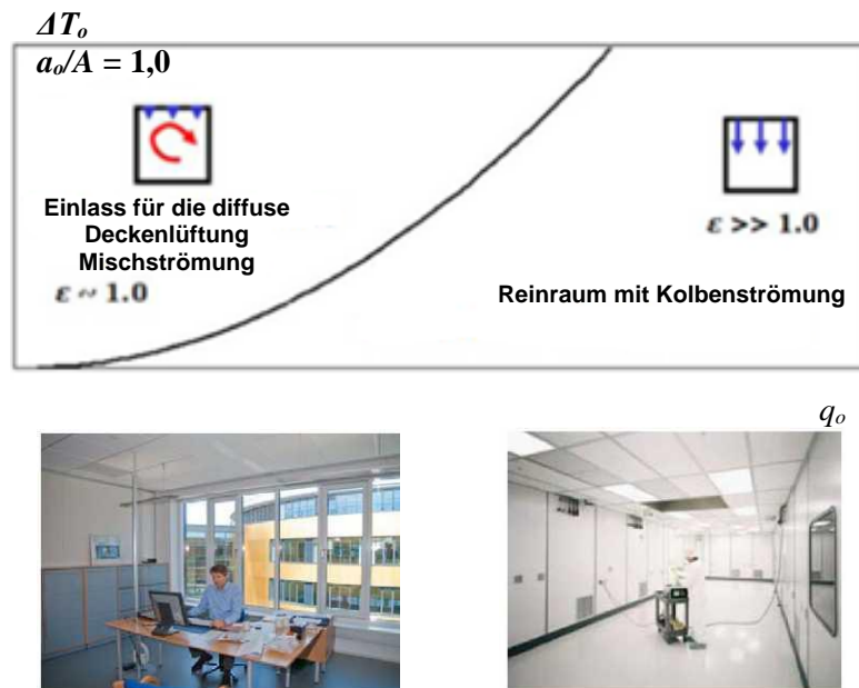
Abbildung 4: q - \Delta T -Diagramm der diffusen Deckenlüftung, zwei Anwendungsbeispiele: Büro und Reinraum [9]
