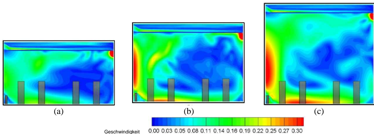
Abbildung 16: Geschwindigkeitsverteilung über die Mittelraumebene bei verschiedenen Raumhöhen. (a) 2,335 m, (b) 3,0 m, (c) 4,0 m [4]
