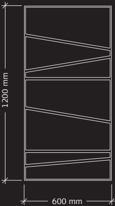
Troldtekt® Tilt Line 7
