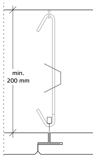
Einbauhöhe, T35-Schienen.
