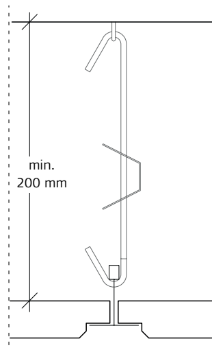
Einbauhöhe, T35-Schienen
