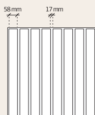
Troldekt® tiles 4 + 4
